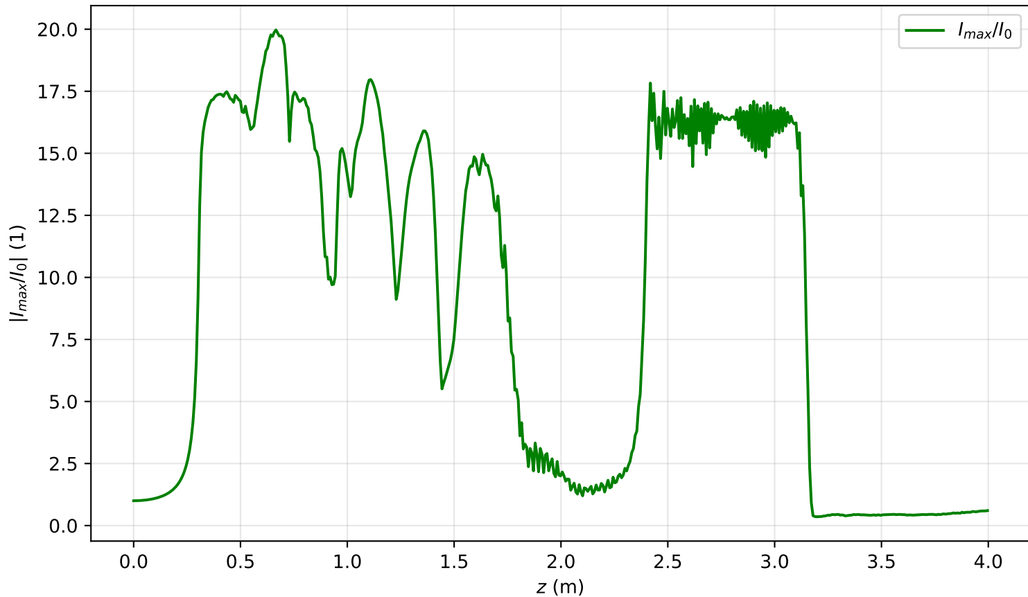
I_{\max}(r=0, z)/I_0 , Pin=9.0Pcr
